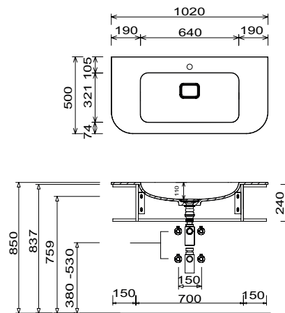
WMS 2610 61 Unterschrankhöhe 240 mm
