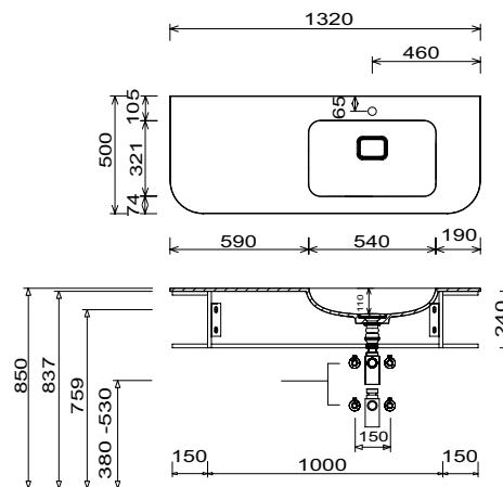
WMS 263L 61 Unterschrankhöhe 240 mm
