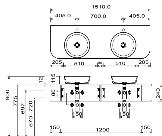
Beispiel Nizza rund Waschtisch Unterschrankhöhe 240 mm
