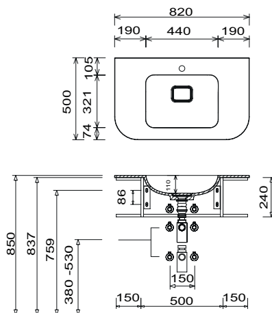
WMS 2608 61 Unterschrankhöhe 240 mm
