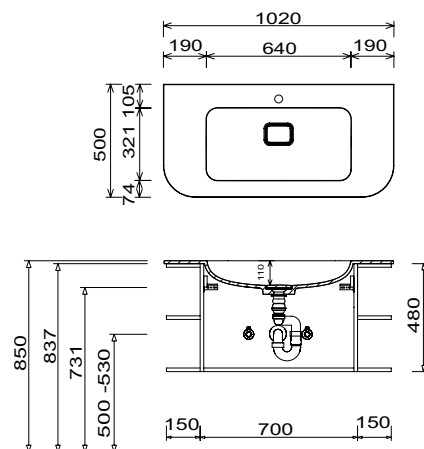
WMS 2610 61 Unterschrankhöhe 480 mm
