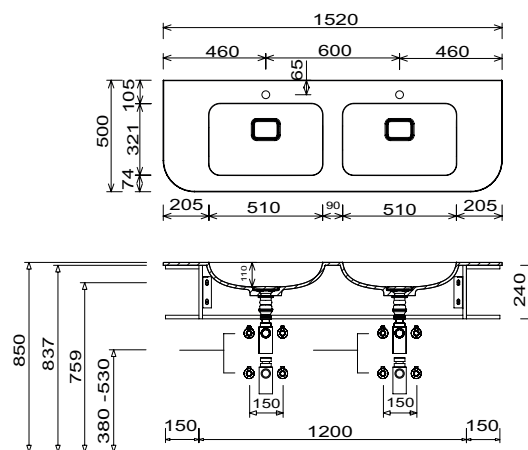
WMS 265D 61 Unterschrankhöhe 240 mm
