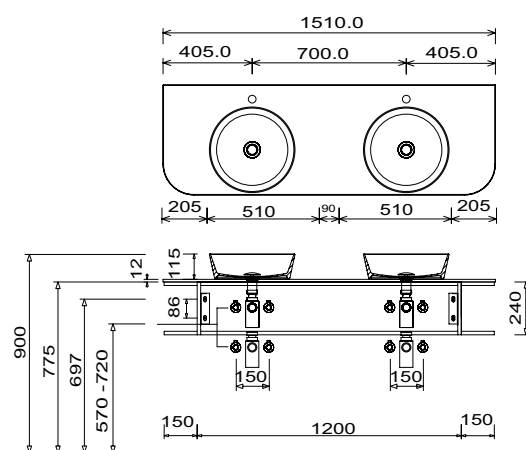
Beispiel Nizza rund Waschtisch Unterschrankhöhe 240 mm
