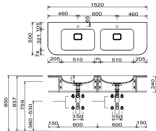
WMS 265D 61 Unterschrankhöhe 240 mm
