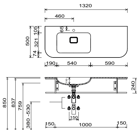
WMS 263R 61 Unterschrankhöhe 240 mm
