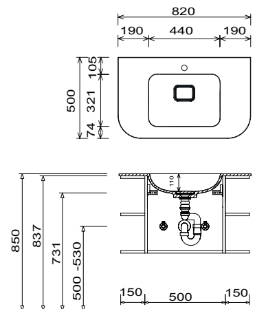
WMS 2608 61 Unterschrankhöhe 480 mm
