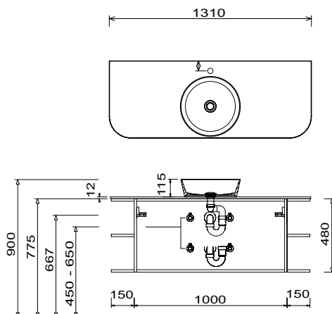
Beispiel Nizza rund Waschtisch Unterschrankhöhe 480 mm
