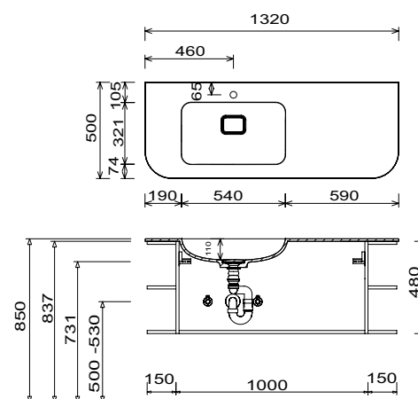
WMS 263R 61 Unterschrankhöhe 480 mm
