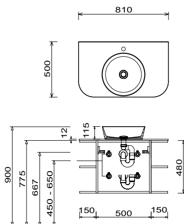
Beispiel Nizza rund Waschtisch Unterschrankhöhe 480 mm
