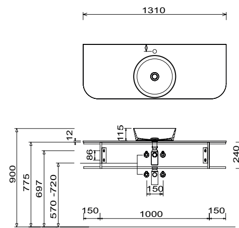
Beispiel Nizza rund Waschtisch Unterschrankhöhe 240 mm
