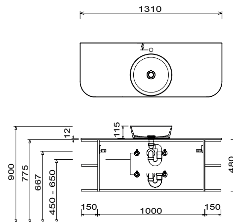
WMS 2613 61 Unterschrankhöhe 480 mm
