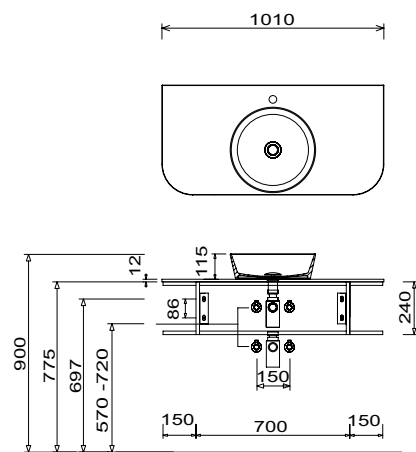
Beispiel Nizza rund Waschtisch Unterschrankhöhe 240 mm
