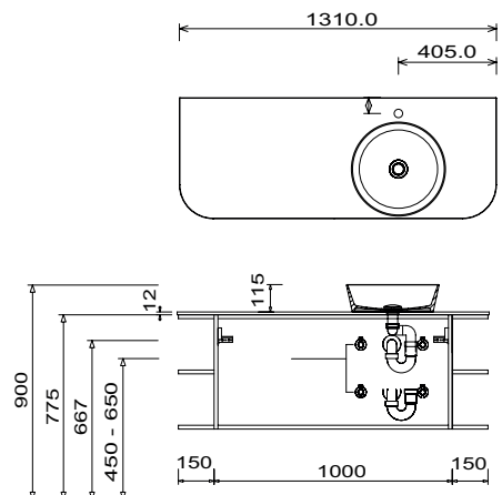
Beispiel Nizza rund Waschtisch Unterschrankhöhe 480 mm
