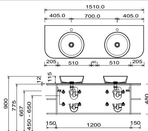
Beispiel Nizza rund Waschtisch Unterschrankhöhe 480 mm
