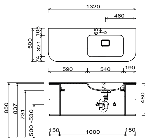
WMS 263L 61 Unterschrankhöhe 480 mm
