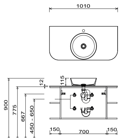
Beispiel Nizza rund Waschtisch Unterschrankhöhe 480 mm
