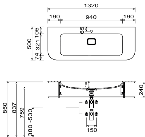
WMS 2613 61 Unterschrankhöhe 240 mm
